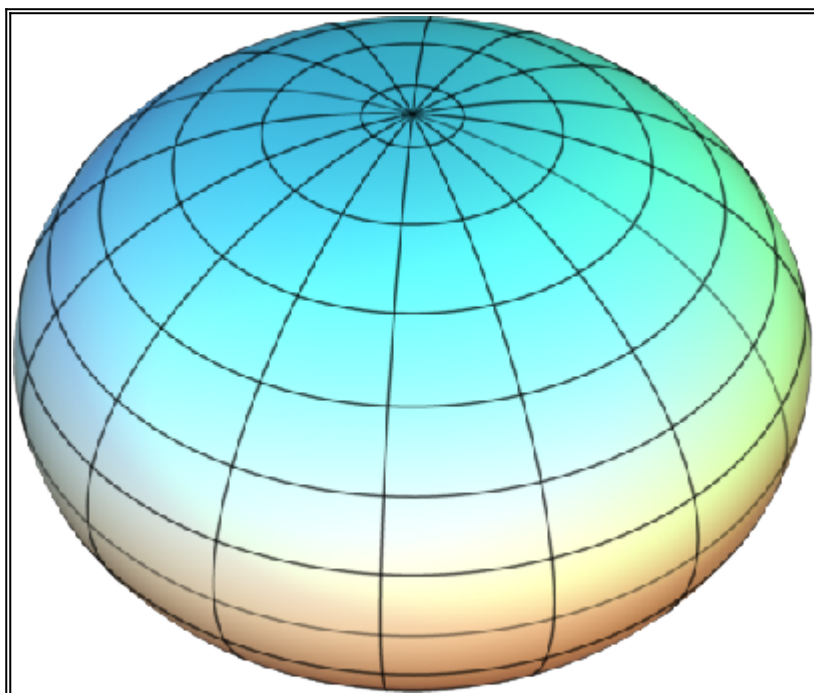
СФЕРОИД
